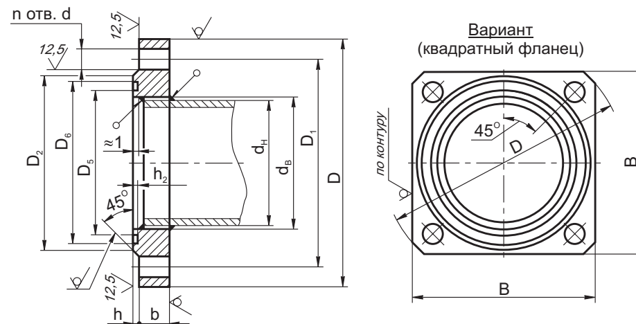
Рис. 4. Фланцы по ГОСТ 33259-2015 (исполнение уплотнительных поверхностей - D)
