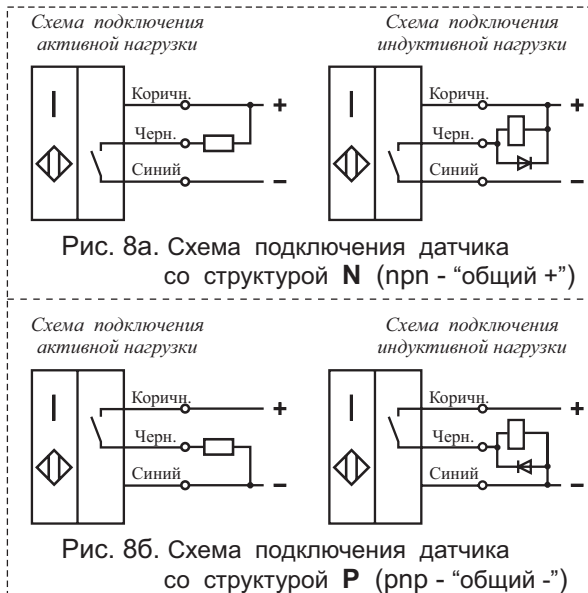
Рис. 8а. Схема подключения датчика со структурой N (npp - "общий +") Рис. 8б. Схема подключения датчика со структурой P (npp - "общий -")
