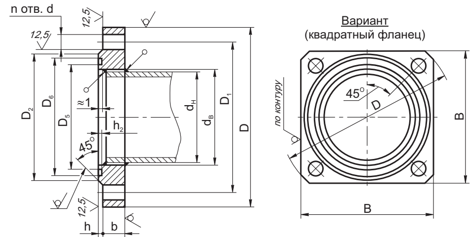
Рис. 4. Фланцы по ГОСТ 33259-2015 (исполнение уплотнительных поверхностей - D)
